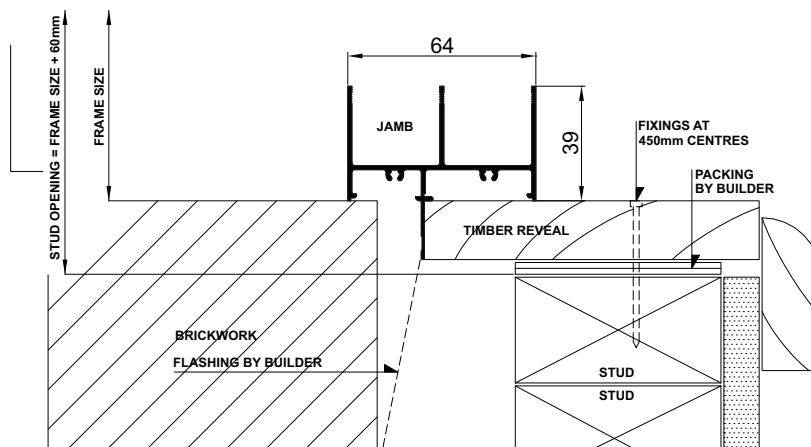
JAMB DETAIL
